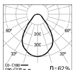
VEGA/E D100 LIGHT+ 4000K HO
