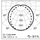
TTP 70 L0620 TOP 4000K LO
