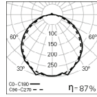
TTP 70 L0620 TUP 4000K HO
